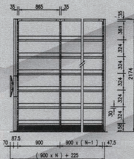
側視圖
